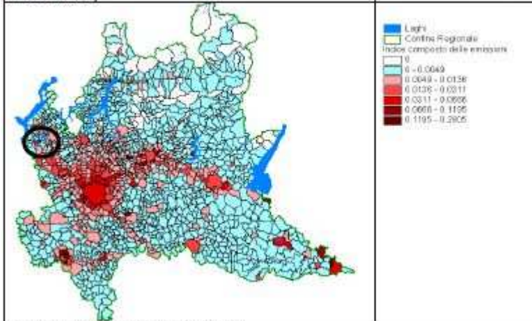
Indicatore composto di qualità dell'aria (Media comunale della somma normalizzata di NOx, PM10, SO2 di ciascuna cella)
